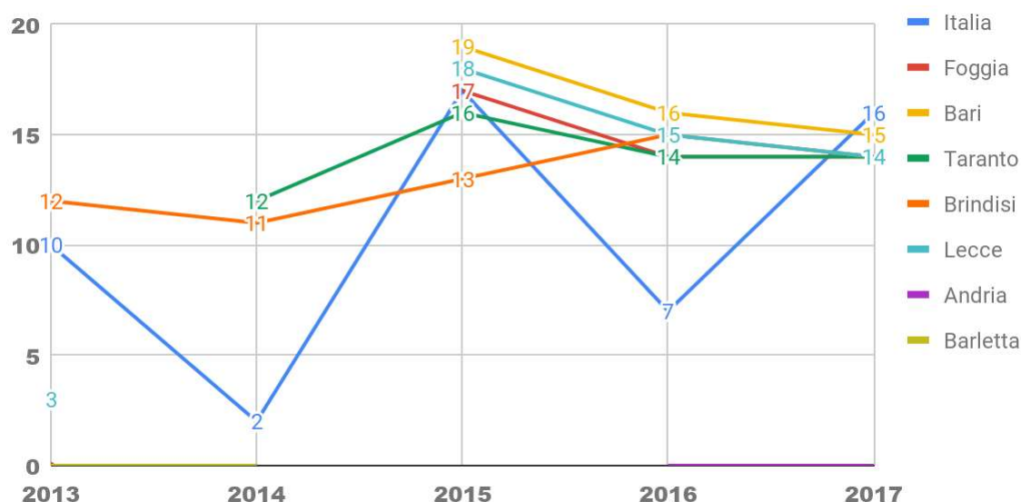
Fig.3.132 - Concentrazione media annuale nei comuni capoluogo di provincia. Puglia, Italia e ripartizioni. Anni 2013-2017 ( \mu\text{g}/\text{m}^3 )
