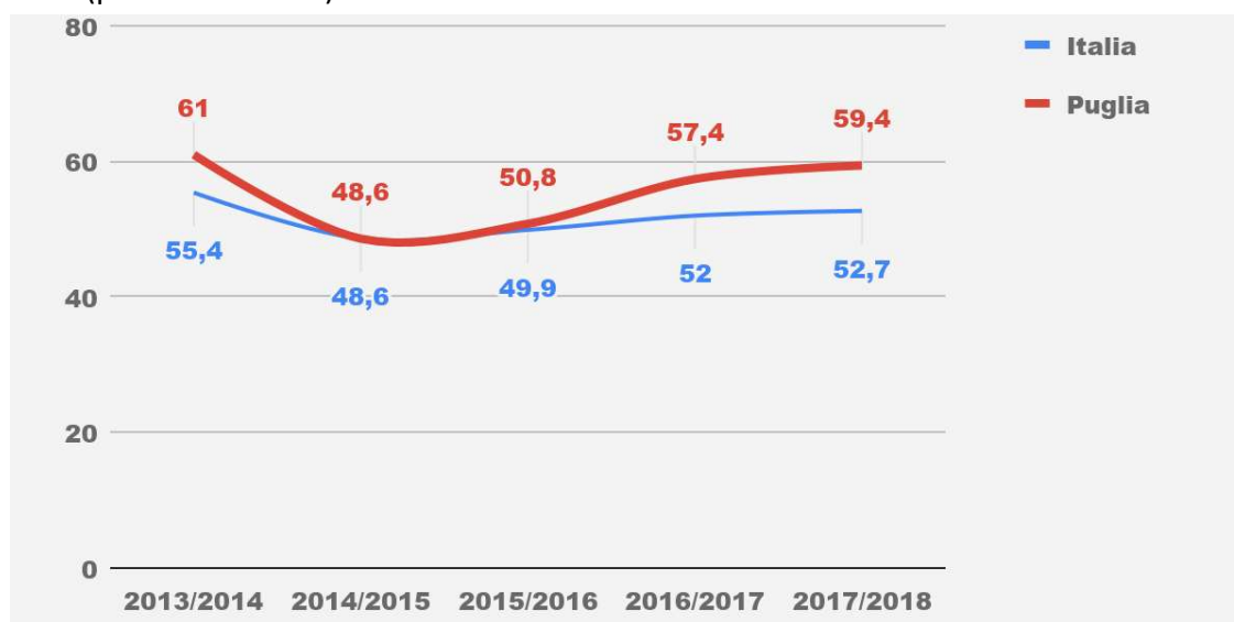
Fig. 3.33 – Copertura vaccinale antinfluenzale età 65+. Puglia, Italia e ripartizioni. Anni 2013-2018 (per 100 abitanti)
