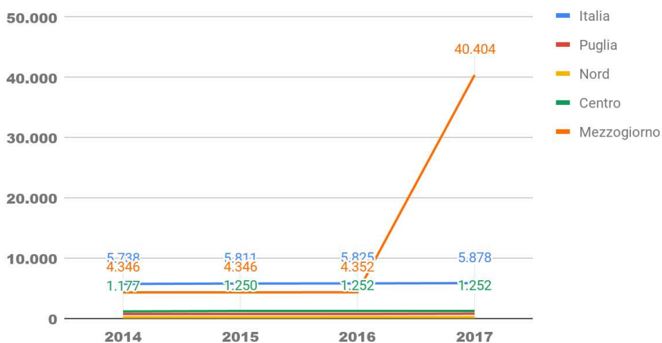
Fig. 3.147 - Aree marine comprese nella rete Natura 2000. Puglia, Italia e ripartizioni. Anni 2014-2017 (kmq)
