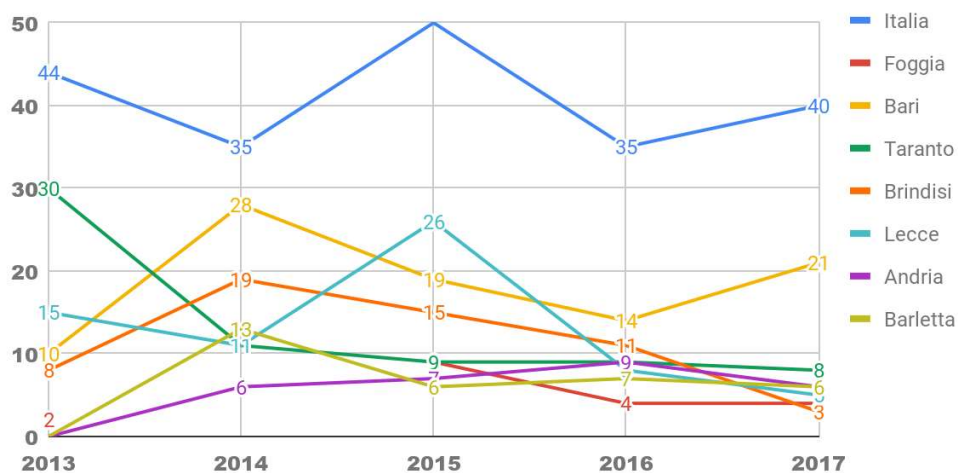
Fig. 3.130 - Superamenti del valore limite giornaliero previsto per il PM10 nei comuni capoluogo di provincia. Puglia, Italia e ripartizioni. Anni 2013-2017 (numero giorni)
