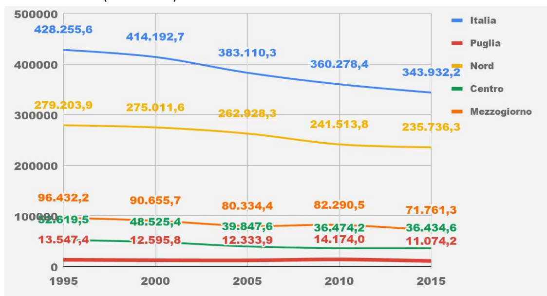
Fig. 3.17 – Emissioni di ammoniaca prodotte dal settore agricolo. Puglia, Italia e ripartizioni. Anni 1995-2015 (tonnellate)
