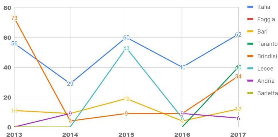
Fig. 3.134 - OZONO n. gg superamento dell'obiettivo nei comuni capoluogo di provincia. Puglia, Italia e ripartizioni. Anni 2013-2017
