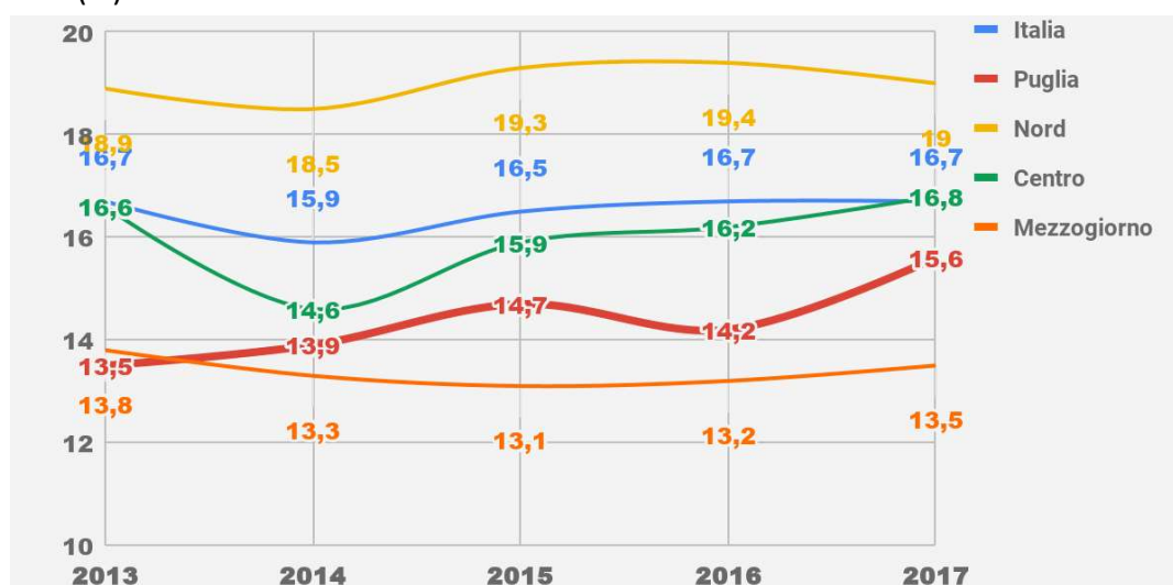
Fig. 3.24 – Alcol puro nella popolazione di 15 anni e più. Puglia, Italia e ripartizioni. Anni 2014-2017 (%)
