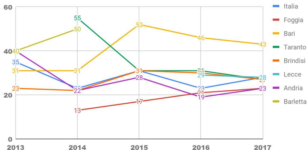
Fig. 3.133 - NO 2 Concentrazione media annuale nei comuni capoluogo di provincia. Puglia, Italia e ripartizioni. Anni 2013-2017 (µg/m 3 )
