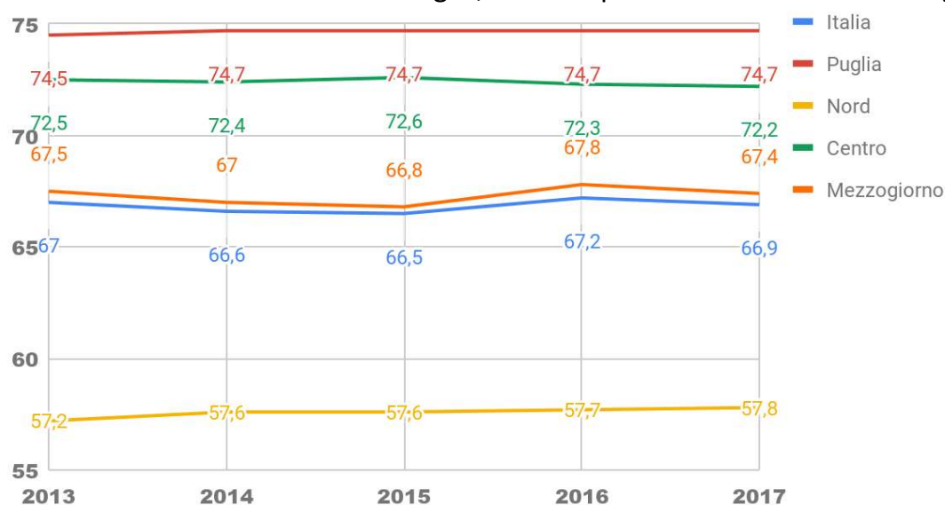
Fig. 3.75 - Coste marine balneabili. Puglia, Italia e ripartizioni. Anni 2013-2017 (%)
