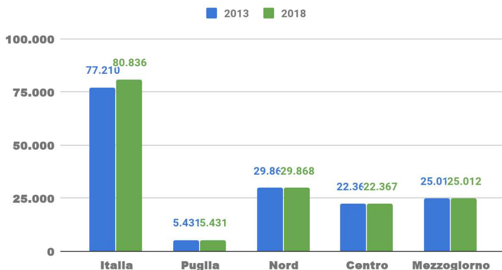
Fig. 3.79 - Zone umide di importanza internazionale (ha). Puglia, Italia e ripartizioni. Anni 2014-2017 (ha)
