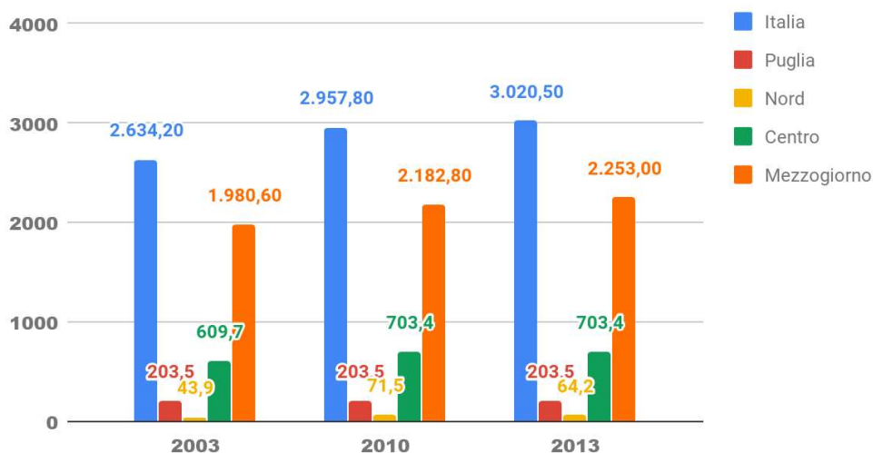
Fig. 3.146 - Aree marine protette EUAP. Puglia, Italia e ripartizioni. Anni 2003, 2010 e 2013 (kmq)
