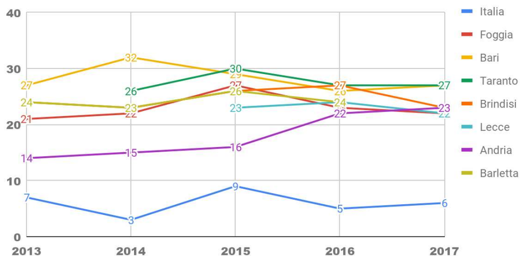
Fig. 3.131 - PM10 Concentrazione media annuale nei comuni capoluogo di provincia. Puglia, Italia e ripartizioni. Anni 2013-2017 ( \mu\text{g}/\text{m}^3 )
