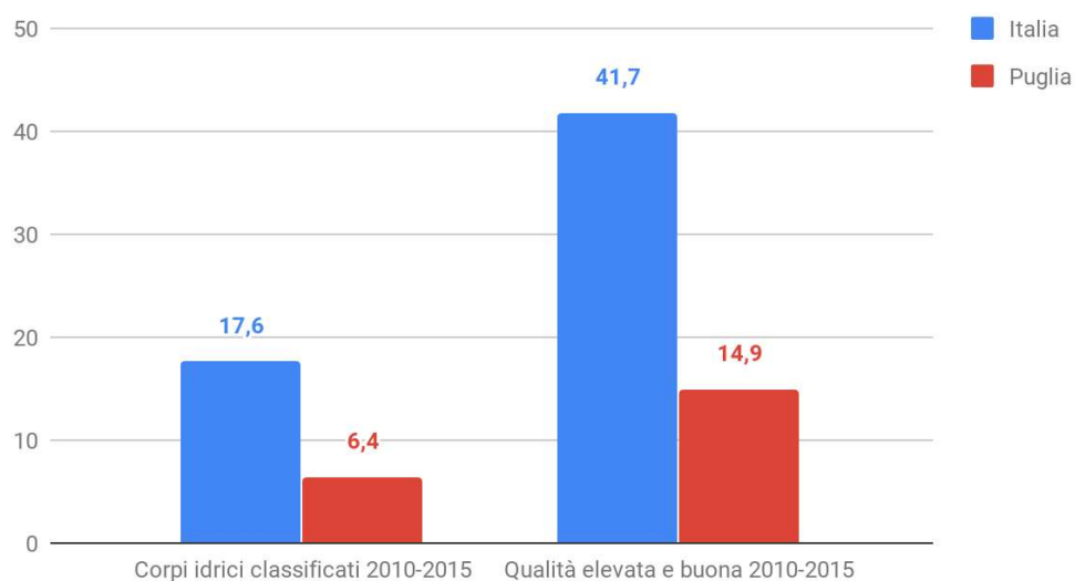
Fig. 3.76 - Corpi idrici in qualità ecologica. Puglia, Italia e ripartizioni. Anni 2010-2015 (%)
