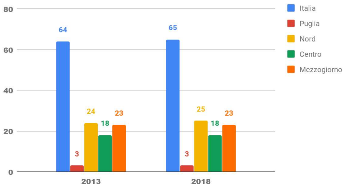
Fig. 3.78 - Numero delle superfici classificate come "zone umide d'importanza internazionale". Puglia, Italia e ripartizioni. Anni 2013 e 2018
