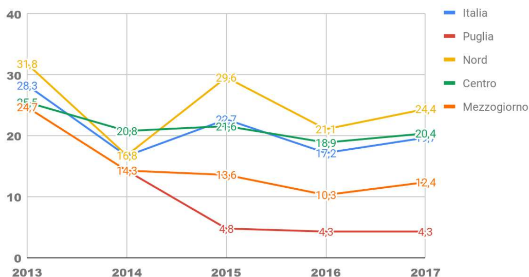
Fig. 3.129 - Qualità dell'aria urbana - Biossido di azoto. Puglia, Italia e ripartizioni. Anni 2013-2017 (%)
